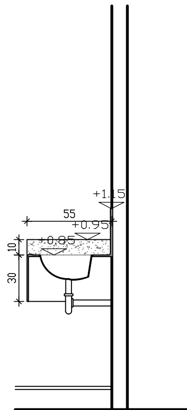
חתך ק.מ. 1:25
